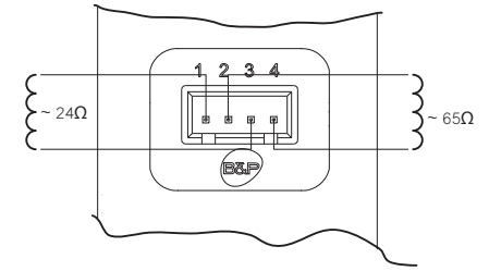
fig. 16 - Connexion soupape de gaz
