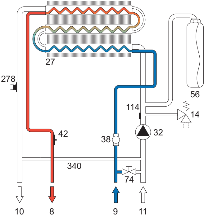
мал. 21 - Гідравлічний контур ГВП
