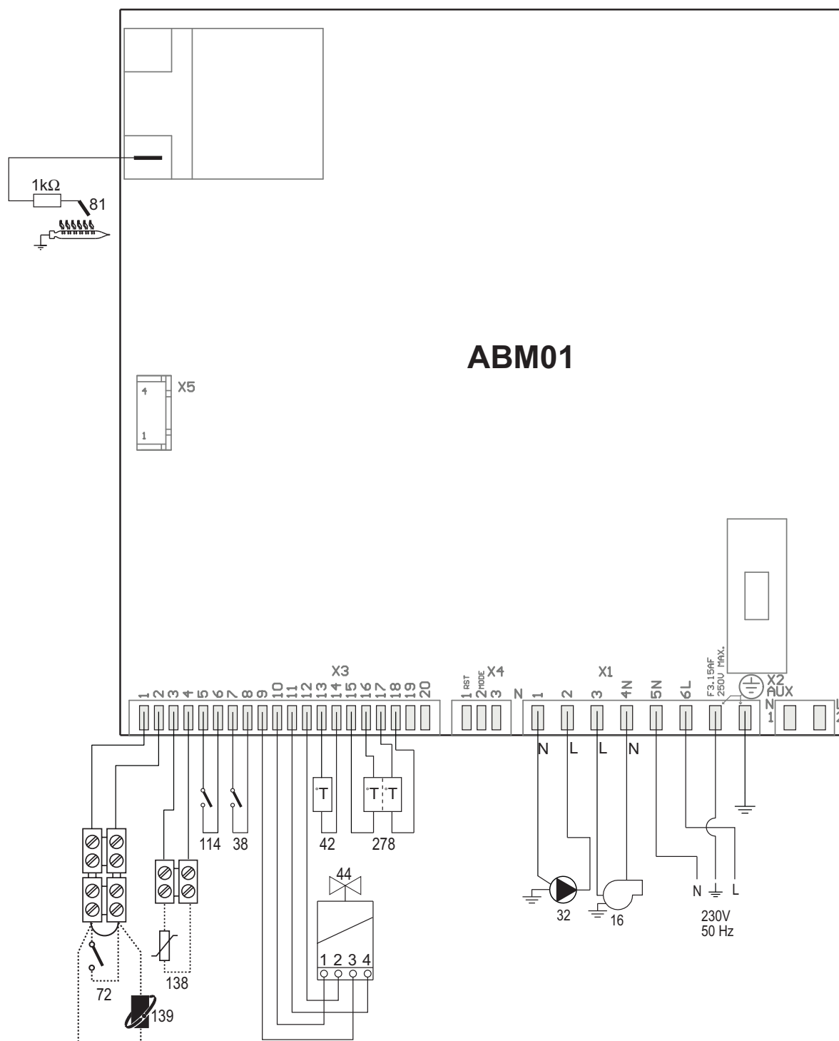
fig. 26 - Circuito elettrico
