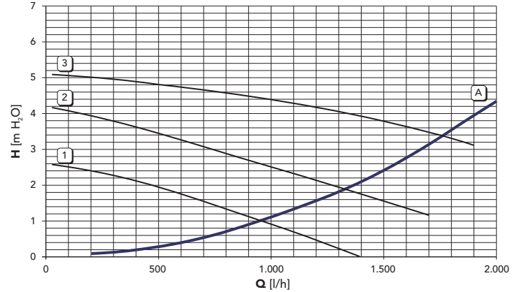
şek. 24 - Sirkülötör yük / basınç kayıpları (DOMItech F 24 D)
