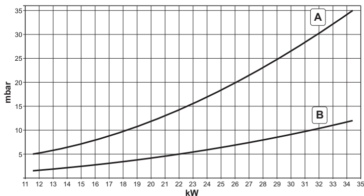
fig. 23 - Diagrama presión - potencia (DOMItech F 32 D)
