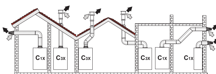
fig. 9 - Esempi di collegamento con tubi coassiali (→ = Aria / → = Fumi)
