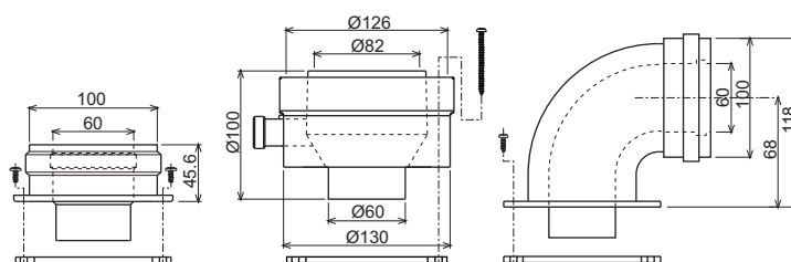
fig. 10 - Accessoires de départ pour conduits coaxiaux
